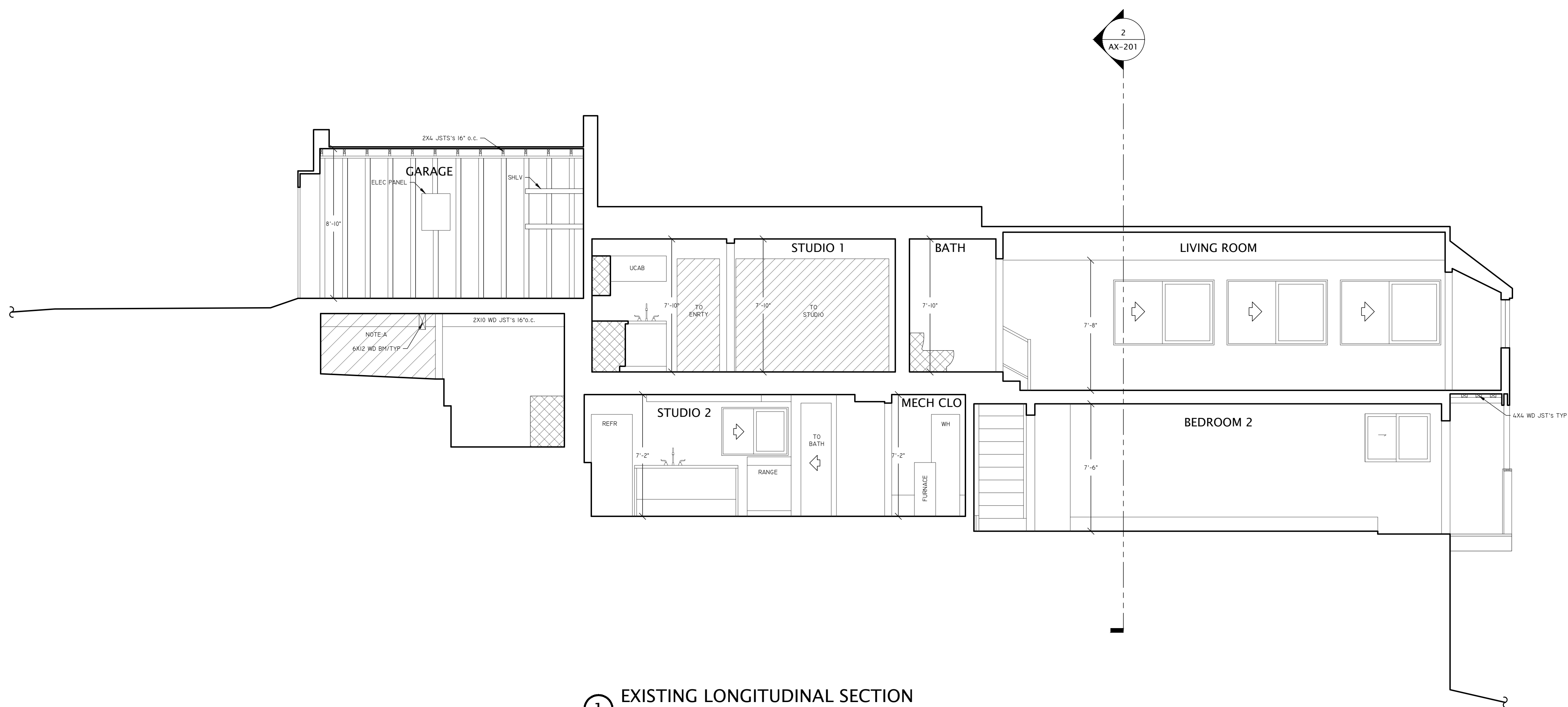
1 EXISTING LONGITUDINAL SECTION
